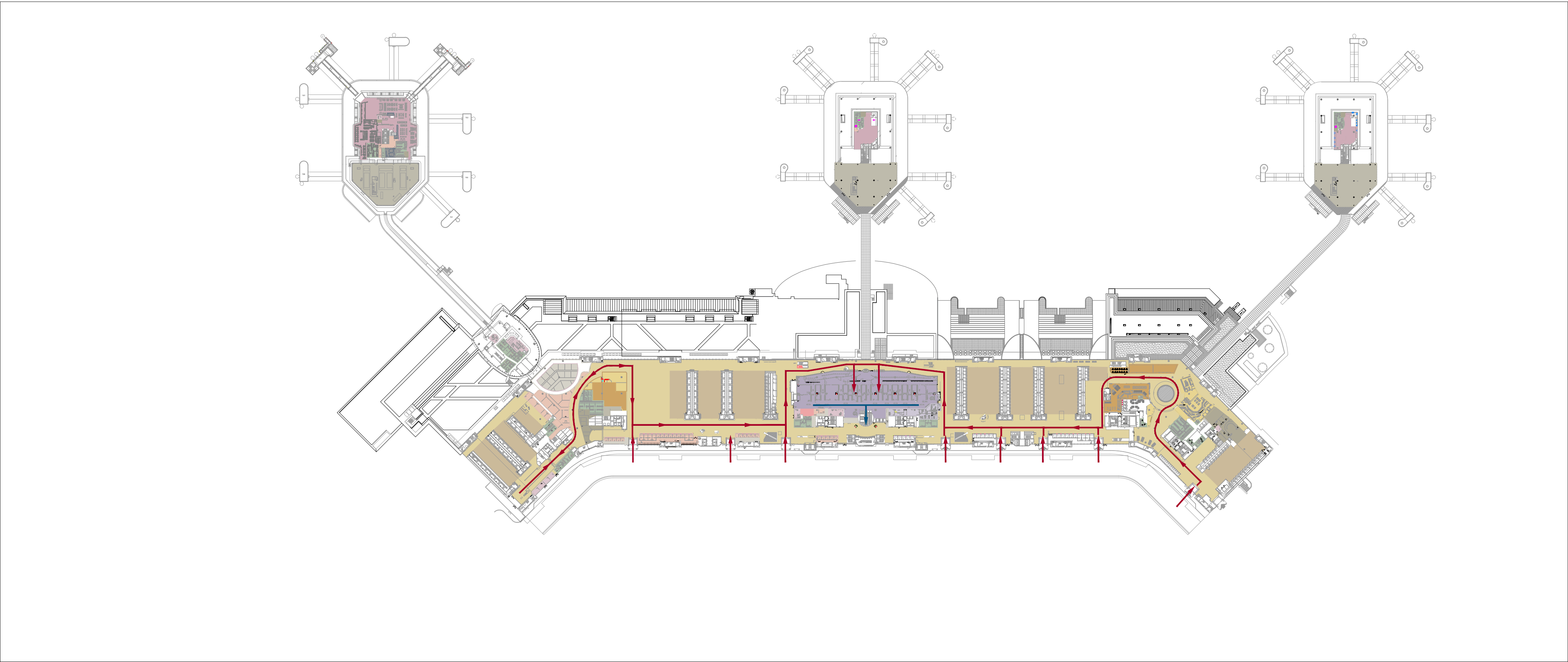
03 Terminal 1 - Pianta piano secondo +14.30 Stato di fatto
