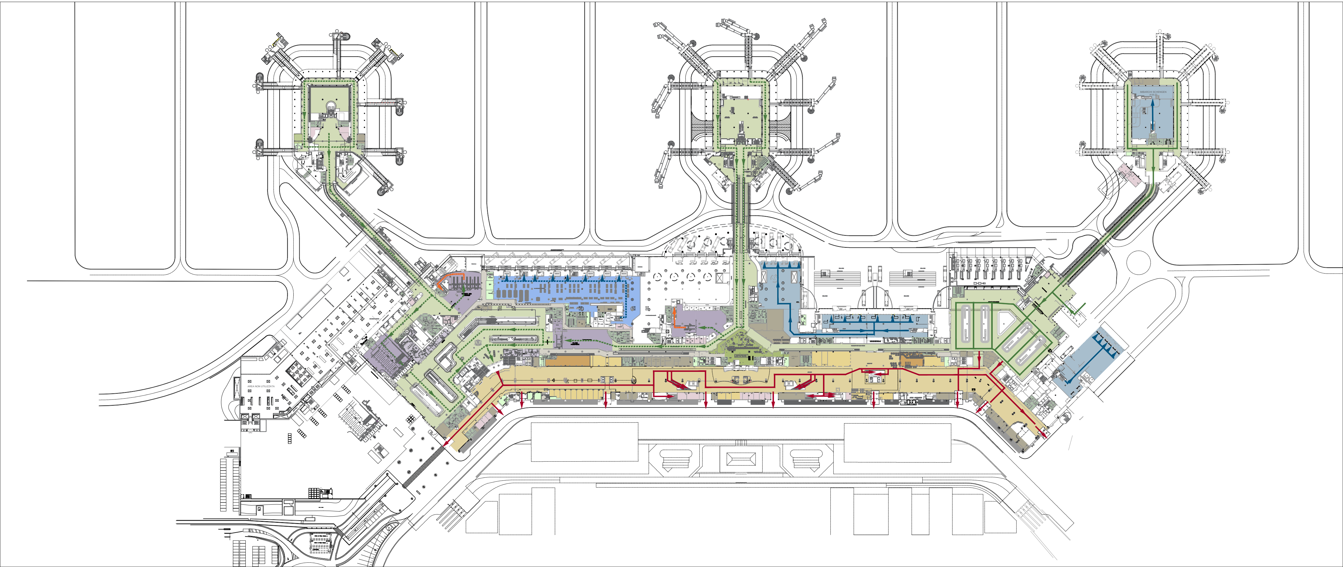
01 Terminal 1 - Pianta piano terra +1.50 Stato di fatto
