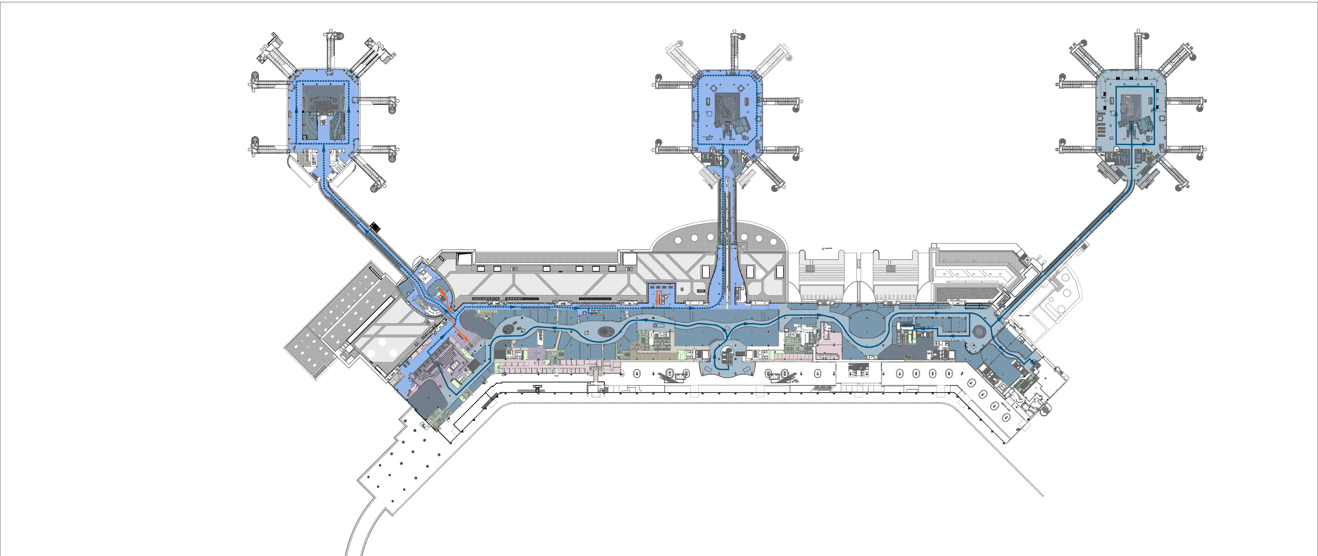
02 Terminal 1 - Pianta piano primo +7.90 Stato di fatto
